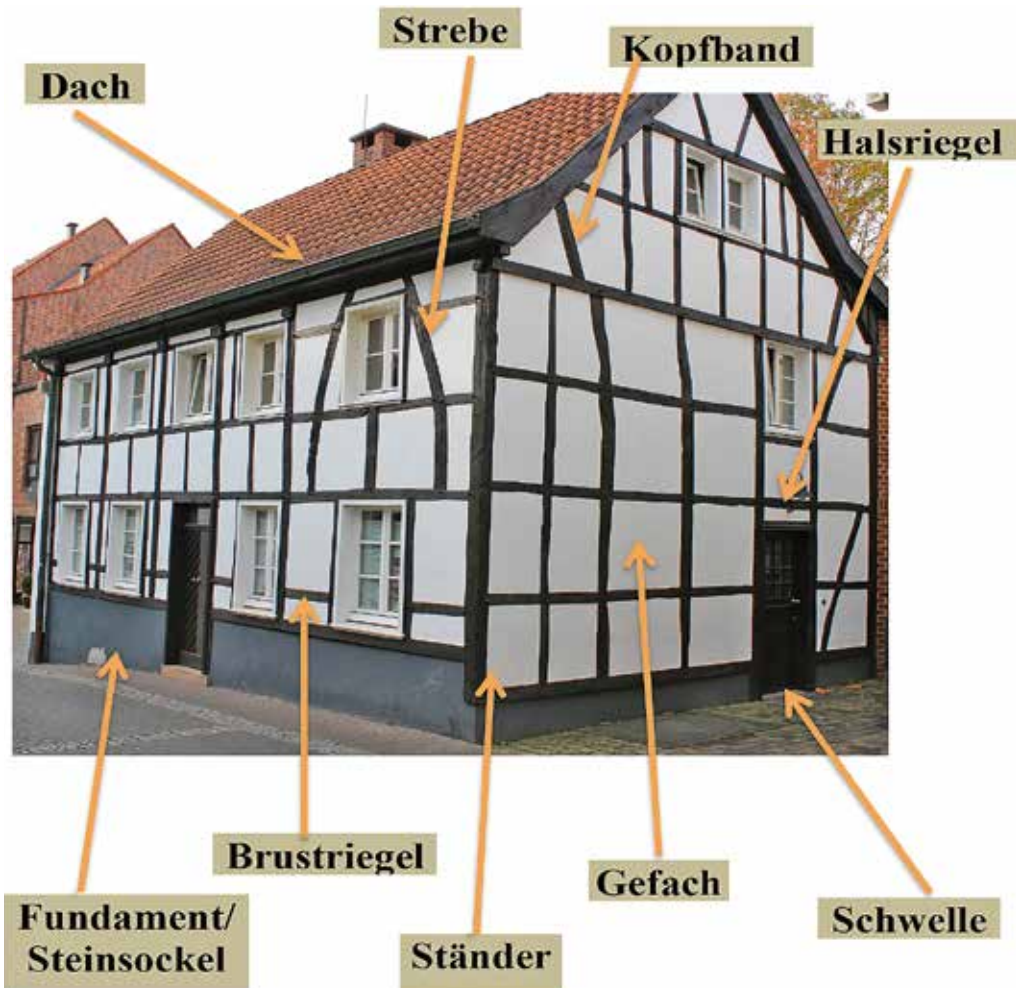
Elemente im Fachwerkbau
